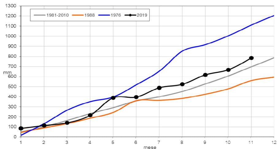
Regione Marche. Andamento della precipitazione cumulata mensile (mm); in nero l'anno attuale, in blu l'anno più piovoso dal 1961, in arancione l'anno meno piovoso dal 1961, in grigio la media 1981-2010
