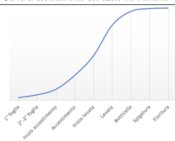
Curva di assorbimento dell'azoto nel frumento
