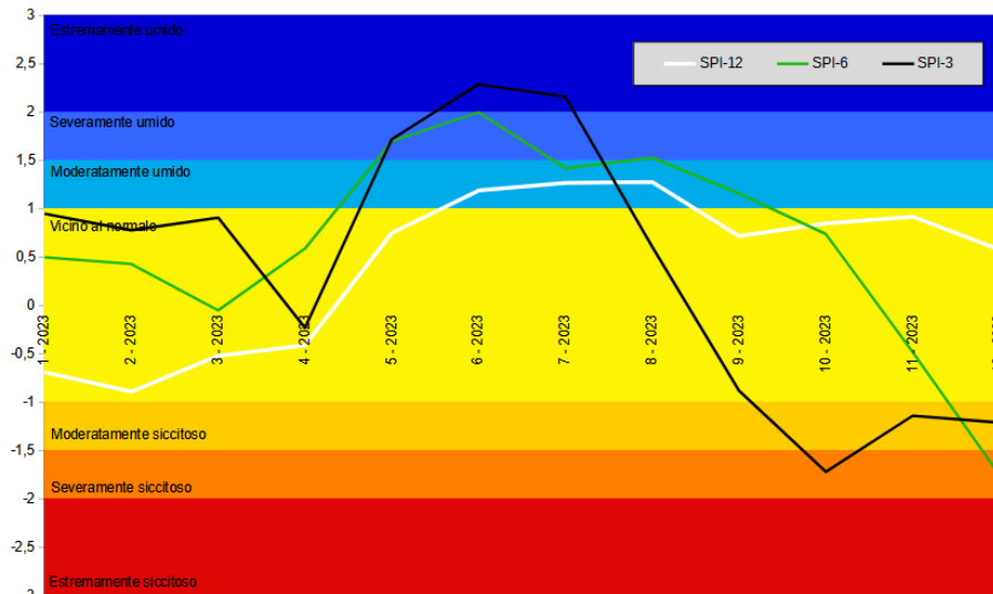
Marche. Andamento mensile indice SPI a 3, a 6 e a 12 mes
