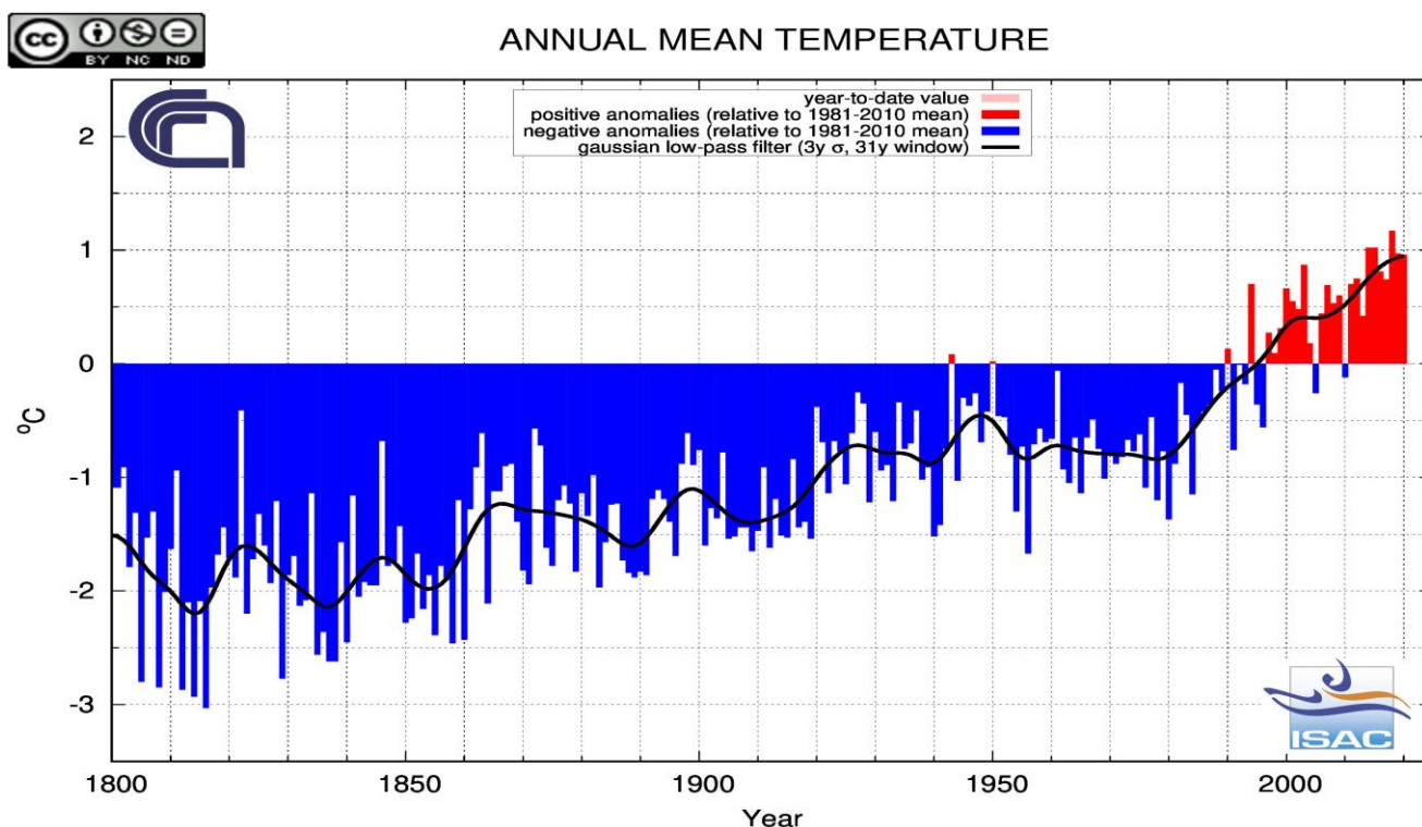
Italia. Andamento anomalia temperatura media annua (°C) 1800-2020 rispetto al 1981-2010 ( fonte )
