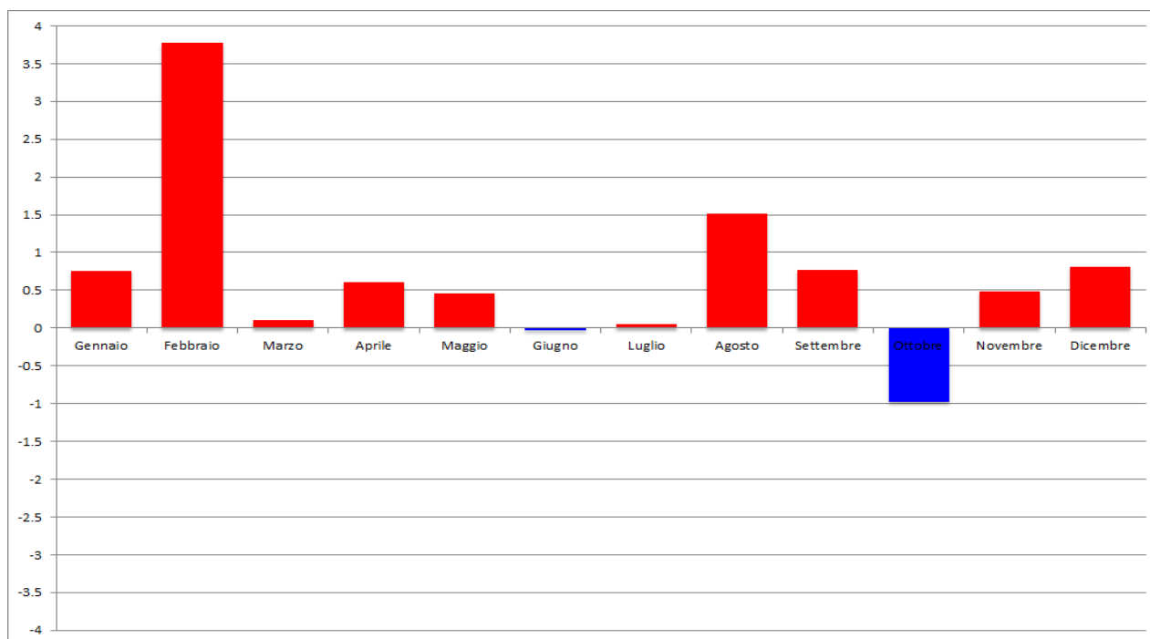
Figura 2. Regione Marche. Anomalia temperatura media mensile (°C) anno 2020 rispetto alla media di riferimento 1981-2010.
