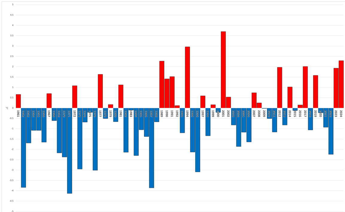
Andamento anomalia della temperatura media regionale del mese di marzo dal 1961 rispetto alla media 1991-2020 (°C). Nell'ultimo decennio, la temperatura media di marzo ha assunto un andamento altalenante intorno alla media. Nel biennio più recente, il 2023-2024, il mese è risultato essere più caldo del normale.
