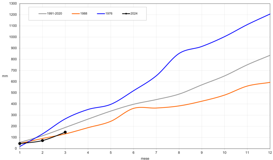
Andamento della precipitazione cumulata mensile (mm); in nero l'anno attuale, in blu l'anno più piovoso (1976) dal 1961, in arancione l'anno meno piovoso (1988) dal 1961, in grigio la media 1991-2020. Nel primo trimestre, il 2024 è in linea con l'anno meno piovoso anche se si osserva un recupero a marzo.
