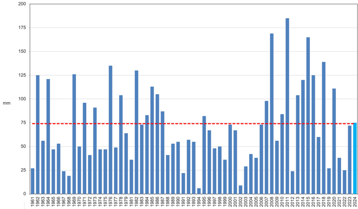
Andamento precipitazione media totale regionale del mese di marzo dal 1961 (mm); la linea tratteggiata rossa rappresenta la media 1991-2020 (mm). La precipitazione di marzo risulta in linea con lo storico.
